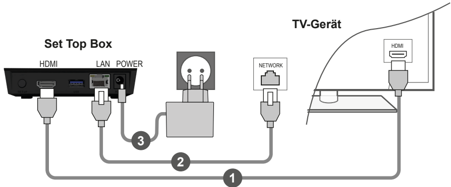
Abbildung 3: Kabelverbindungen
